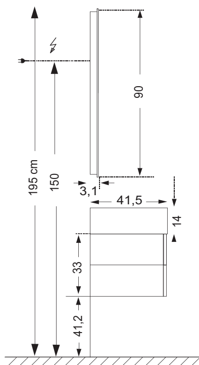
miroir + sous table 2 façades Unterschrank mit 2 Fronten + Spiegel
