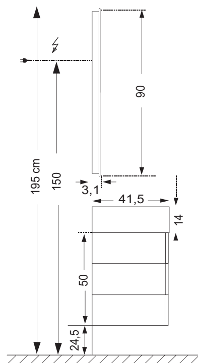
miroir + sous table 3 façades Unterschrank mit 3 Fronten + Spiegel
