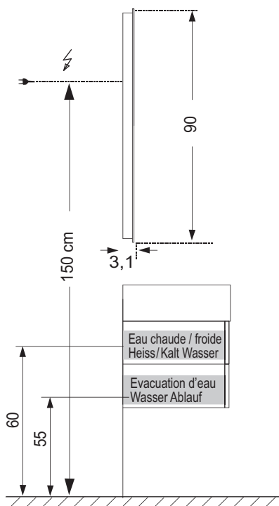
miroir + sous table Unterschrank + Spiegel
